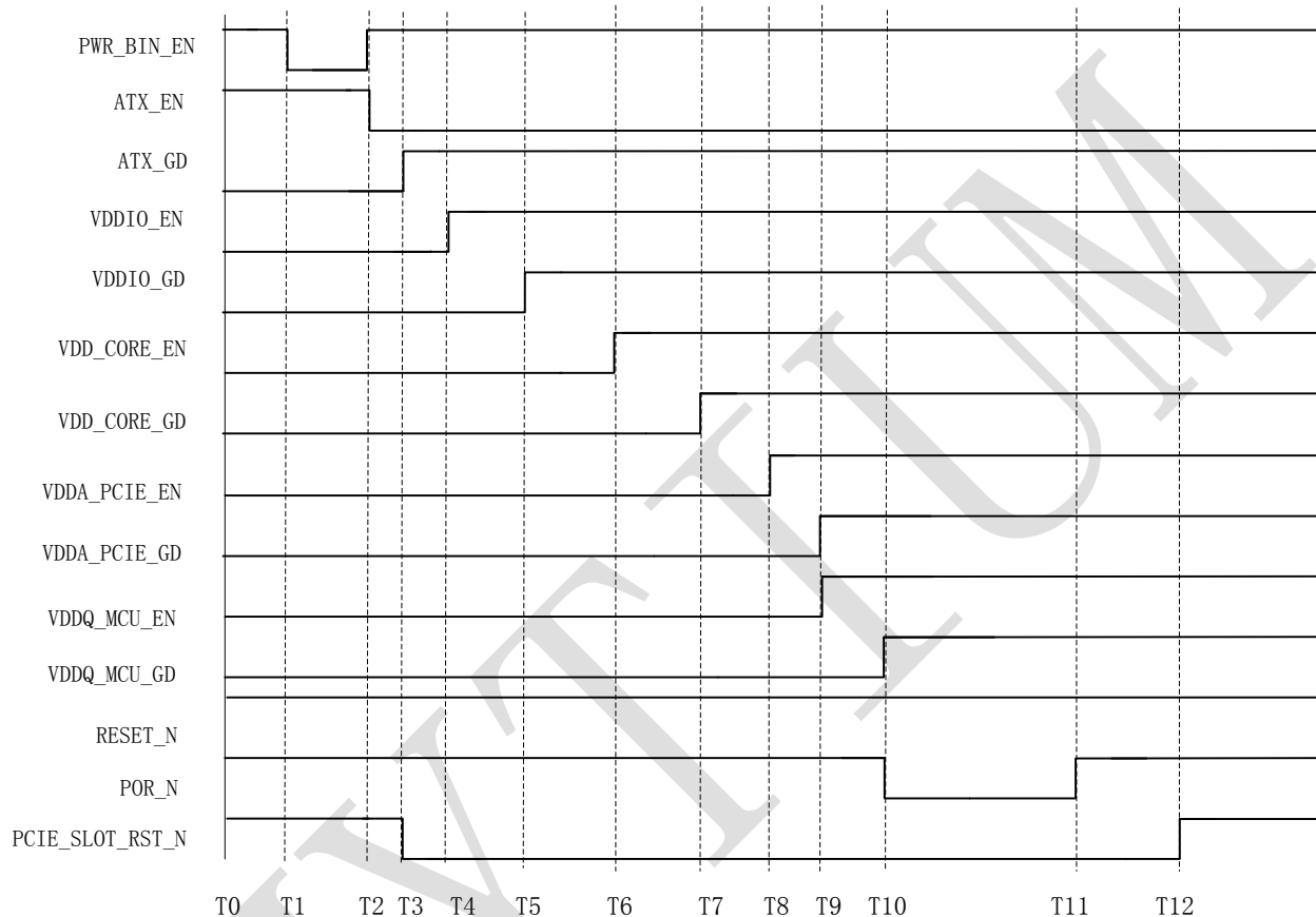
图 3-1 上电复位参考时序图
